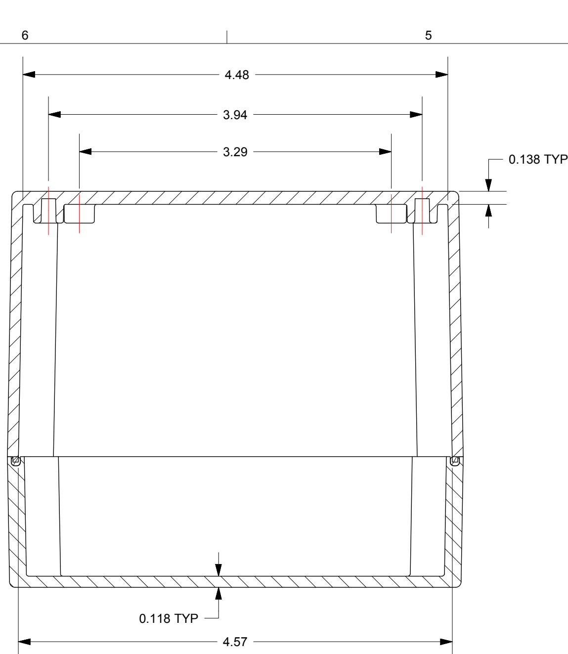
SECTION A-A
