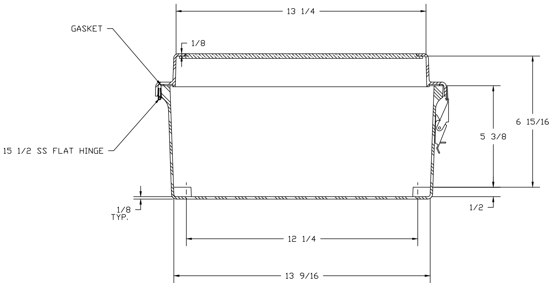
SECTION A-A
