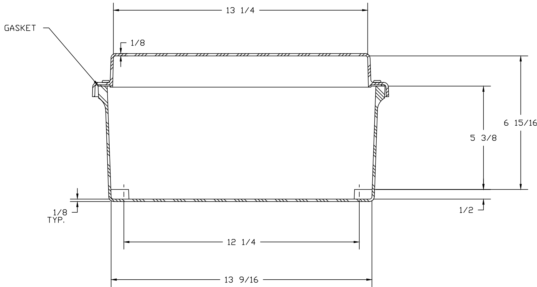
SECTION A-A
