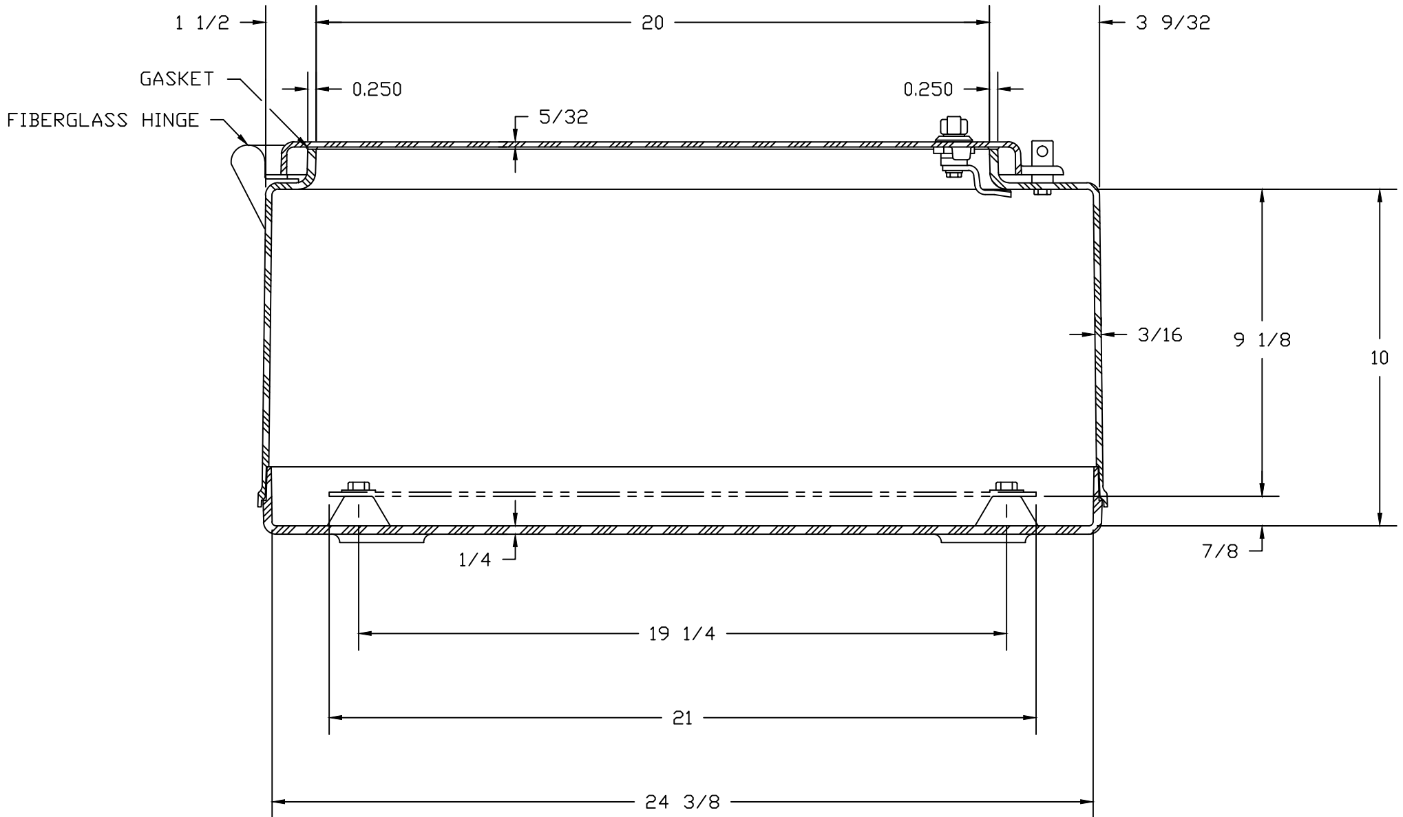
SECTION A-A
