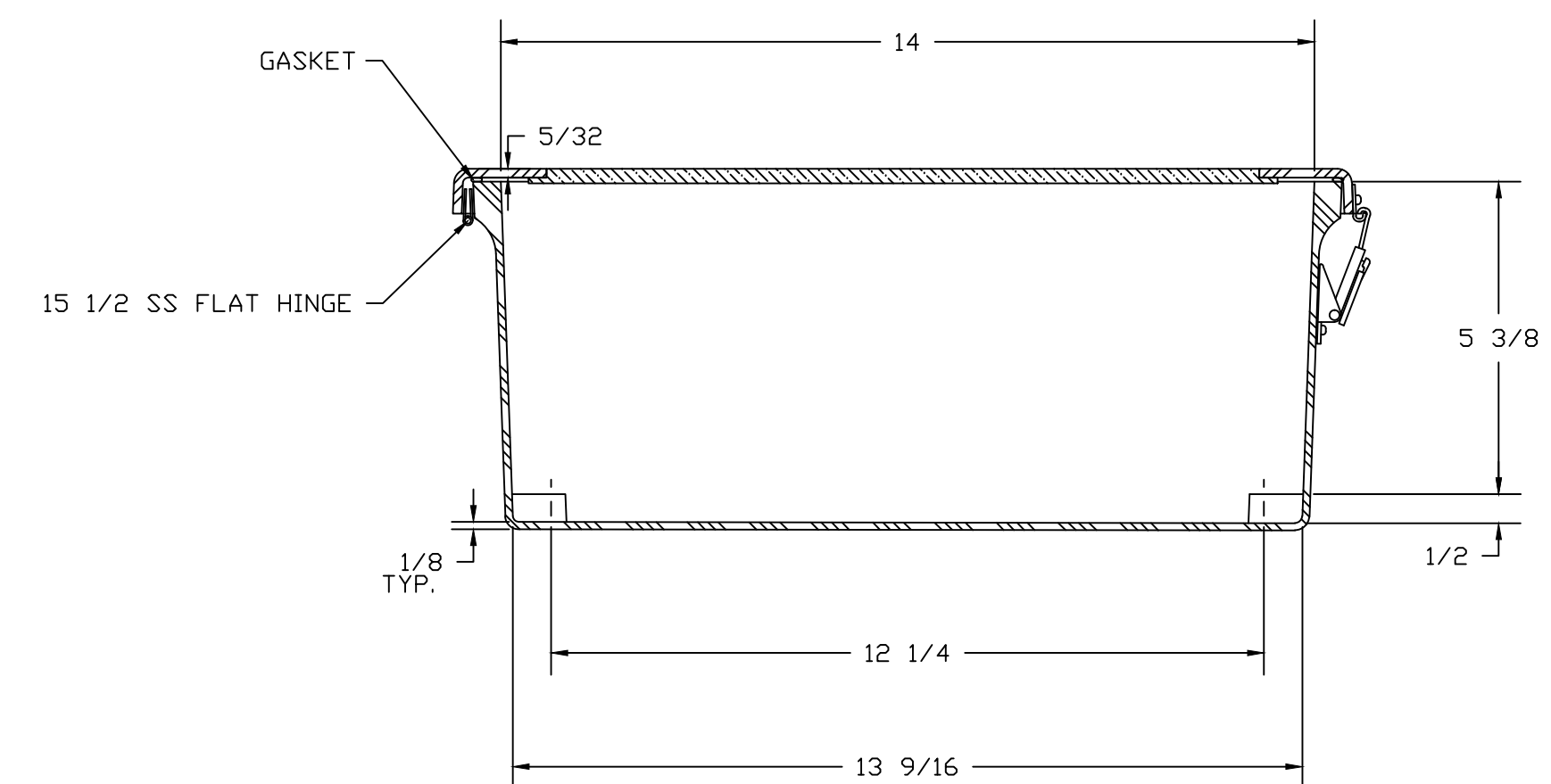
SECTION A-A
