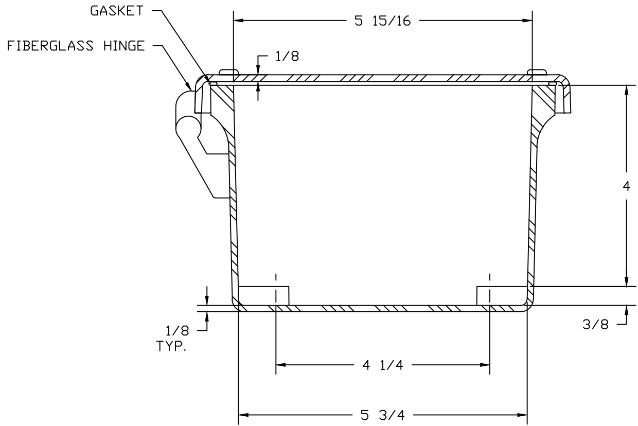
SECTION A-A
