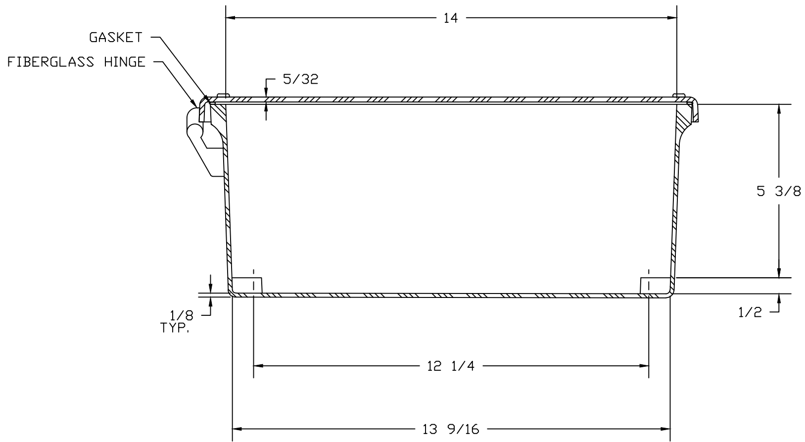
SECTION A-A
