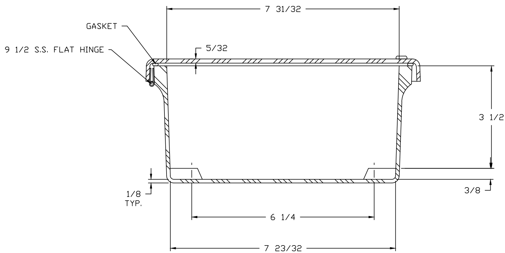
SECTION A-A
