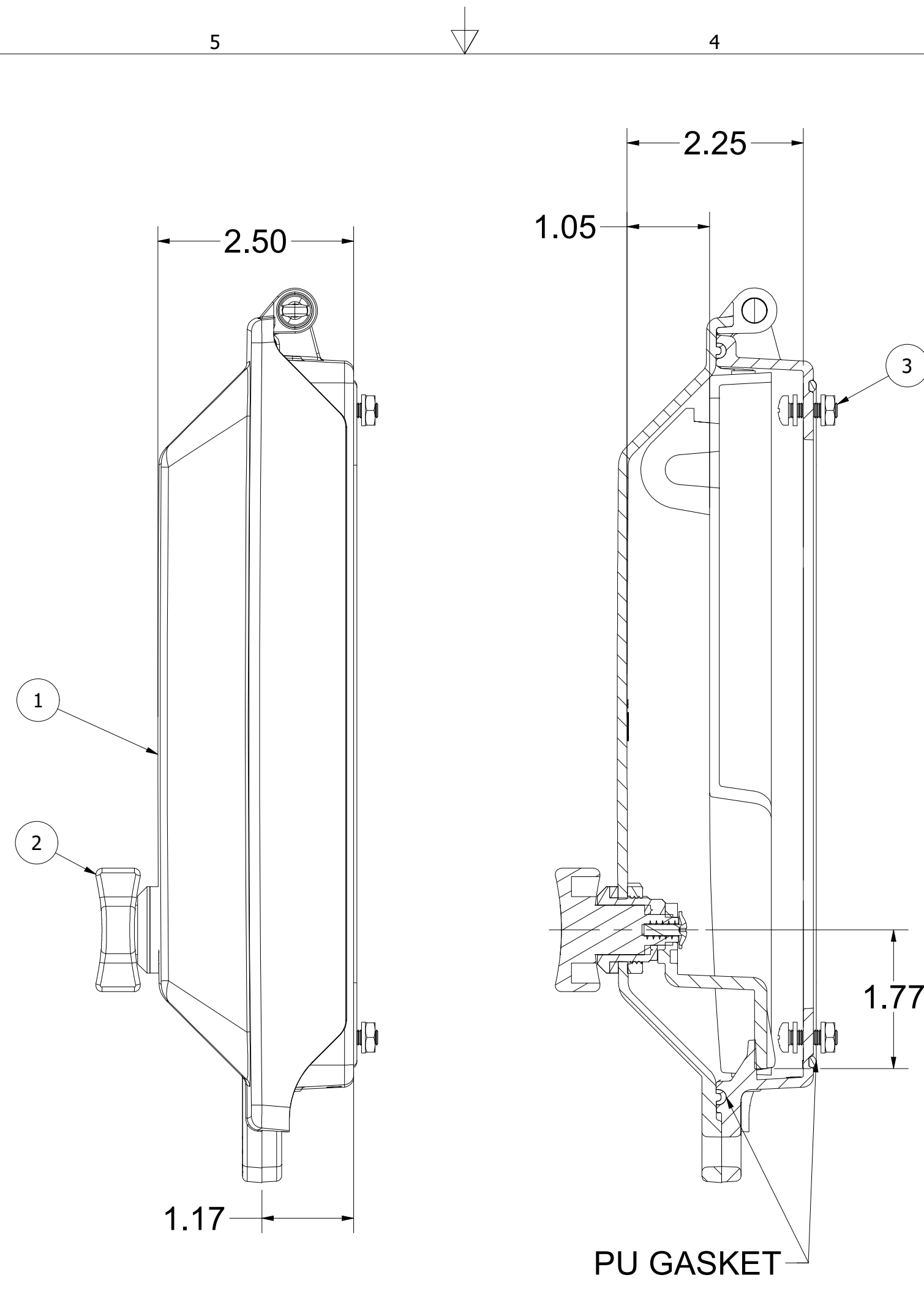
SECTION A-A
