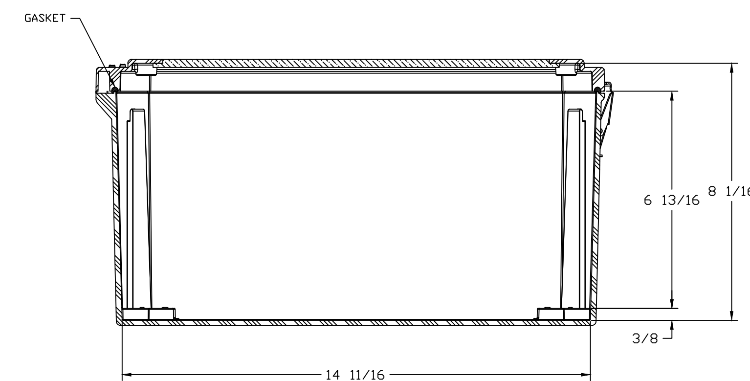
SECTION A-A
