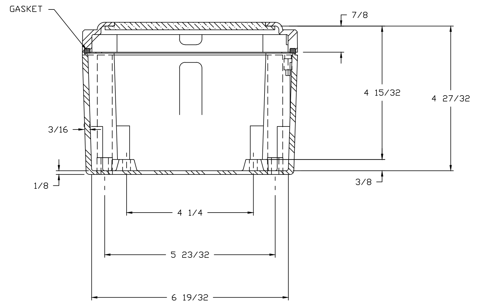
SECTION A-A
