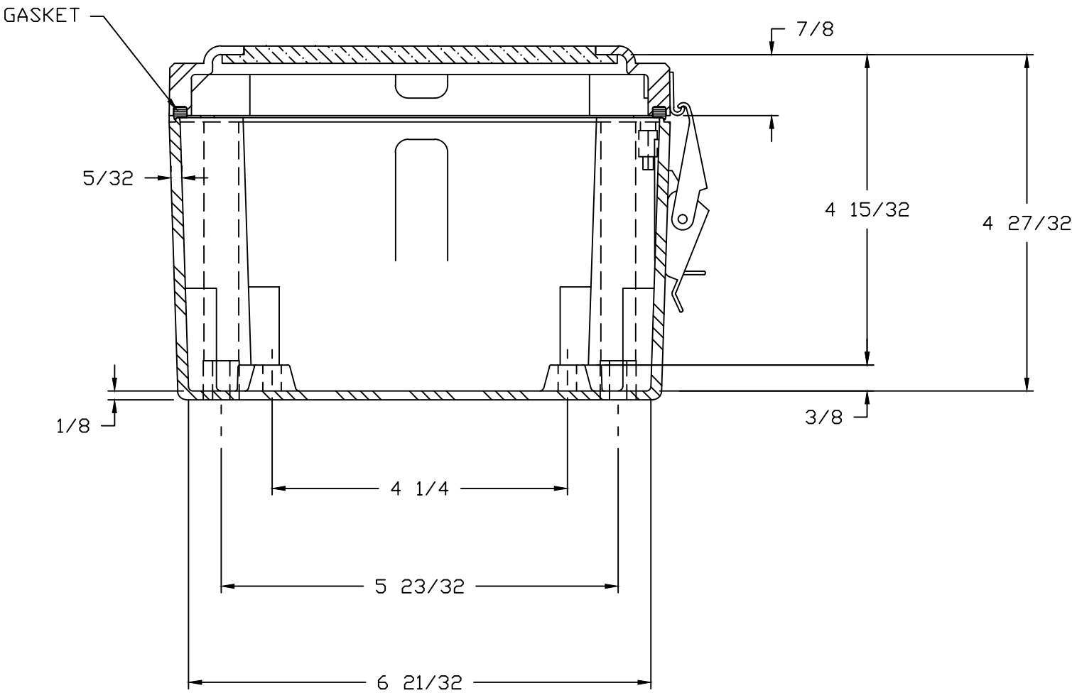
SECTION A-A
