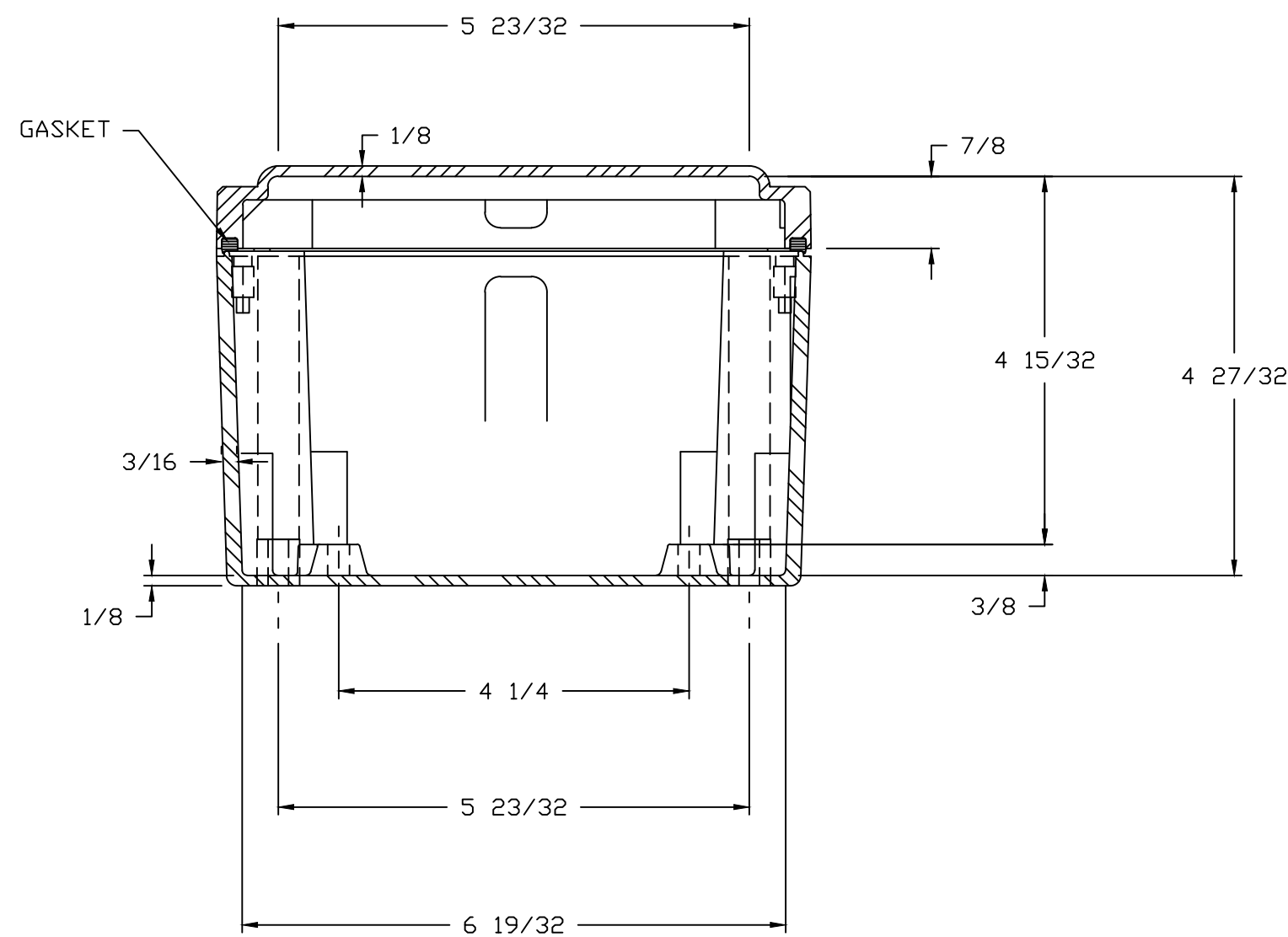
SECTION A-A
