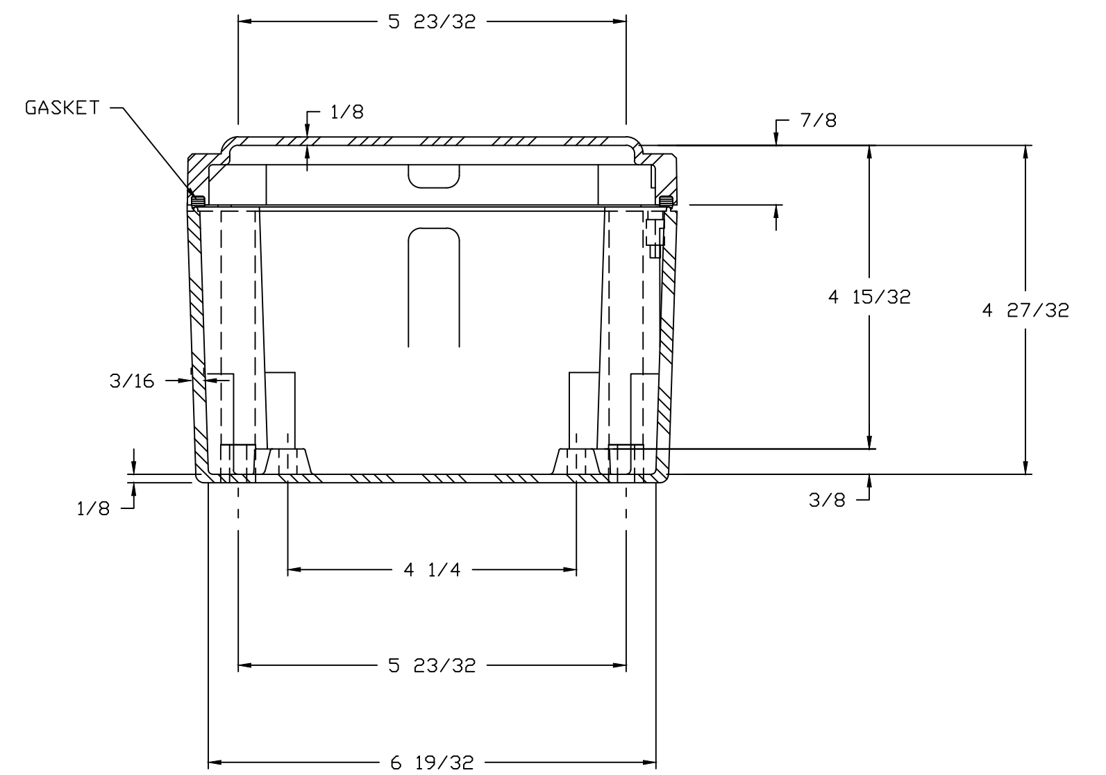
SECTION A-A
