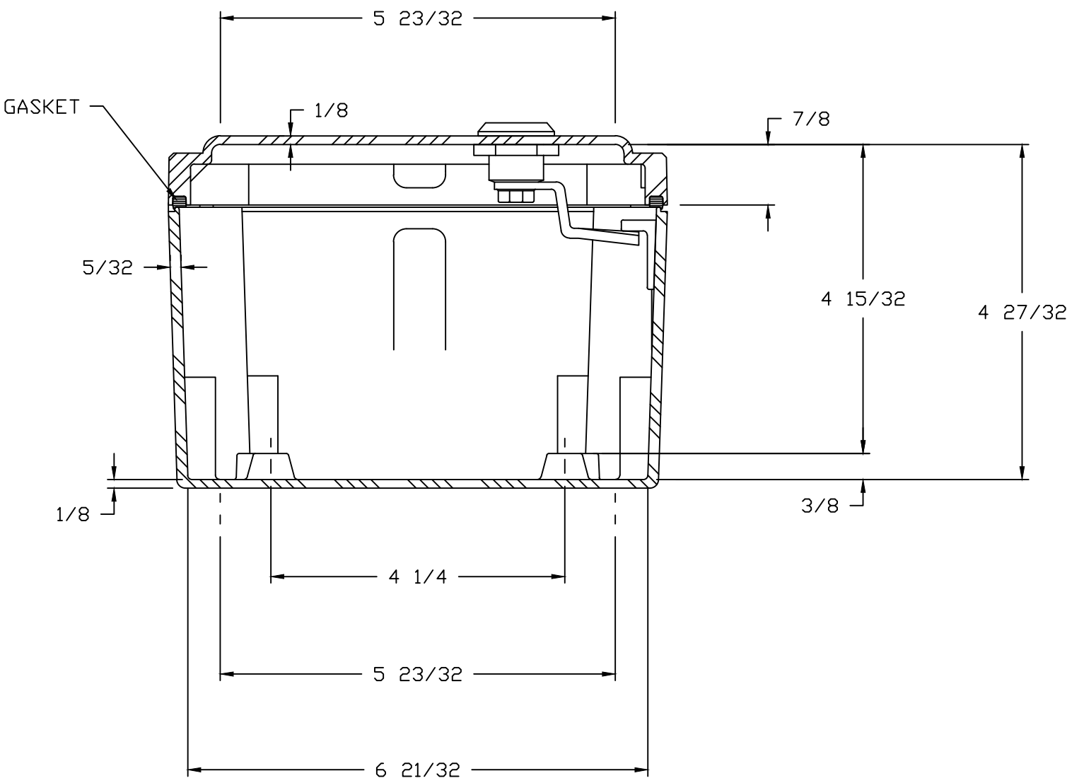
SECTION A-A
